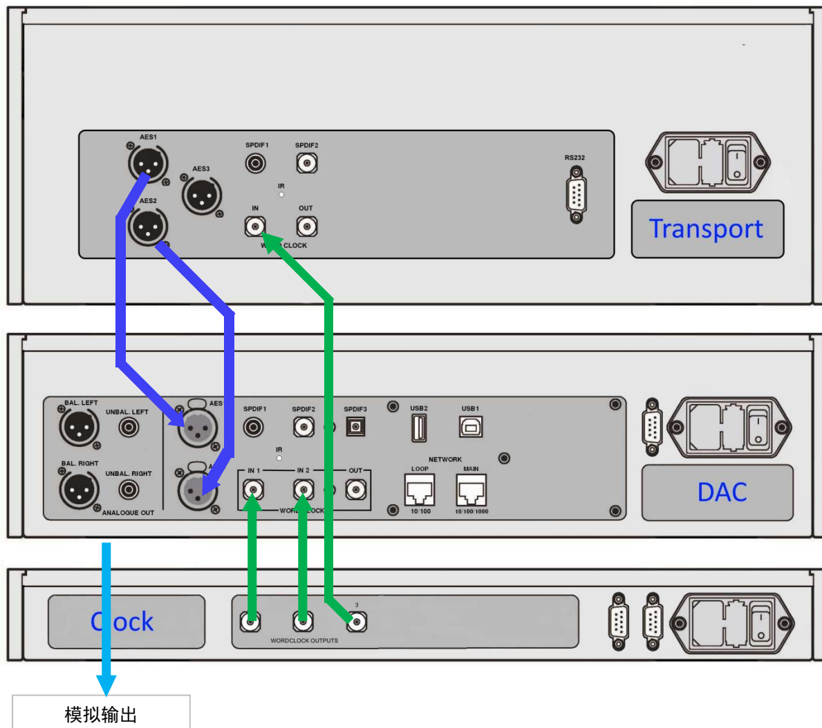
图 7 - 将 Rossini DAC 和 Clock（音频时脉校准机）与 Transport（CD/SACD 转盘激光唱机）一起使用
