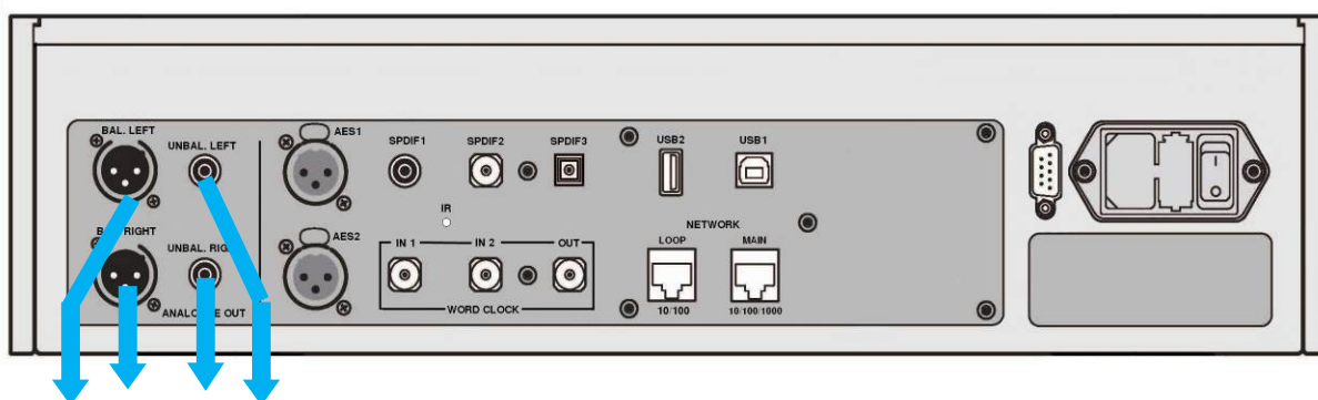
图 1 - Rossini DAC 的基本设置
