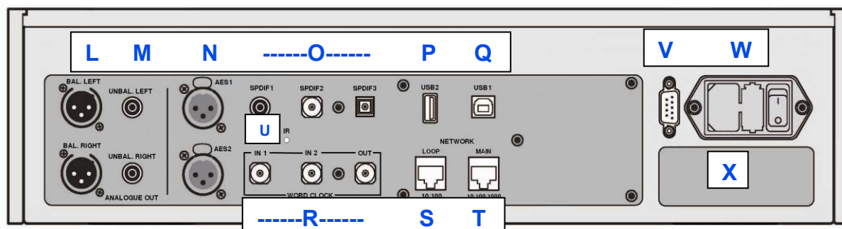
图 9 - 后面板
