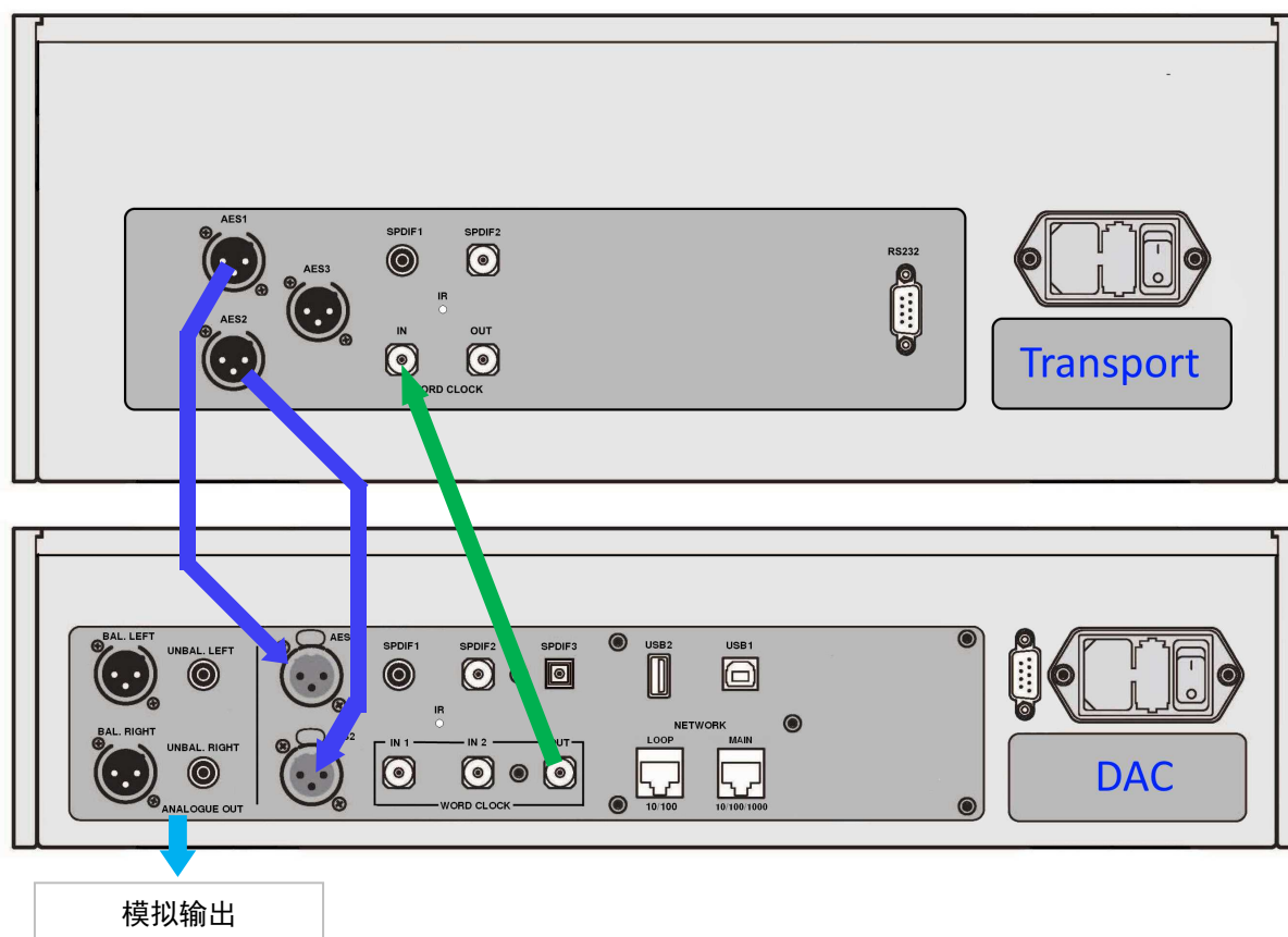
图 6 - 在主模式下将 Rossini DAC 与 Transport (CD/SACD 转盘激光唱机) 一起使用
