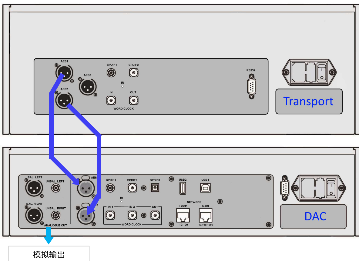
图 3 – 将 Rossini DAC 与 Rossini Transport（CD/SACD 转盘激光唱机）一起使用
